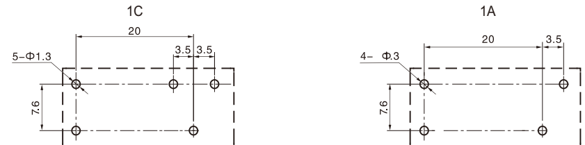
1组-安装孔尺寸 (底视图)
