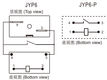
接线图 Wiring Diagram (底视图 Bottom view)
