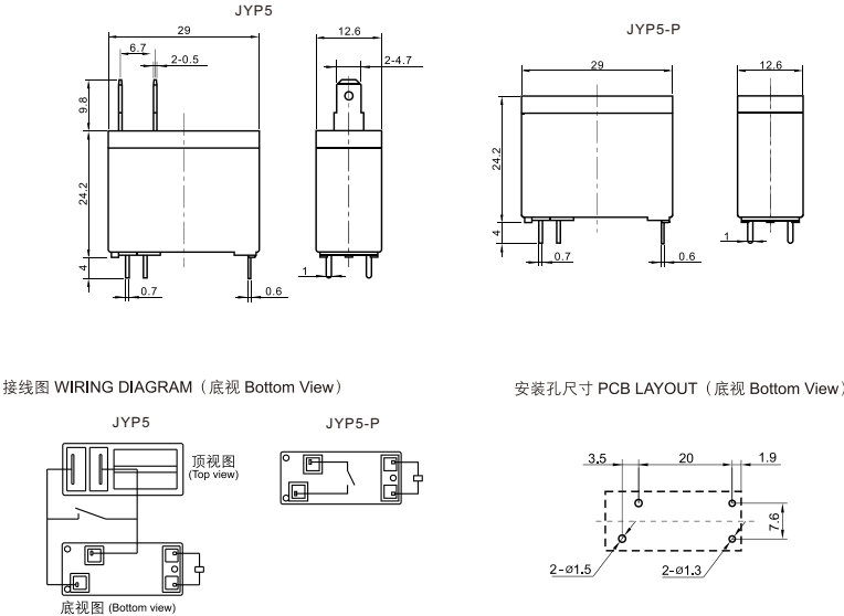
外形尺寸 OUTLINE DIMENSIONS
